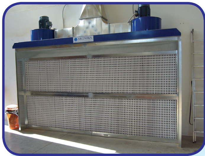
Cabina per verniciatura con aspirazione a secco, con moduli filtranti a fisarmonica.
